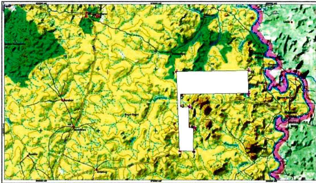
Figure : Carte de localisation du Permis de recherche « Ouest Kolia ».
