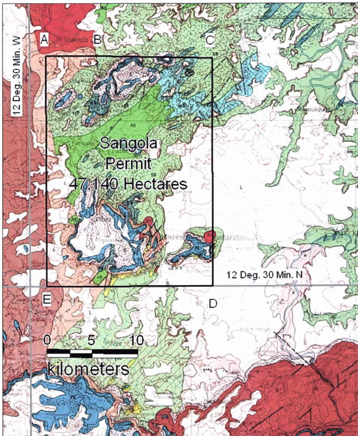
Extrait de la Carte géologique au 1/200 000, feuille de Kédougou.
